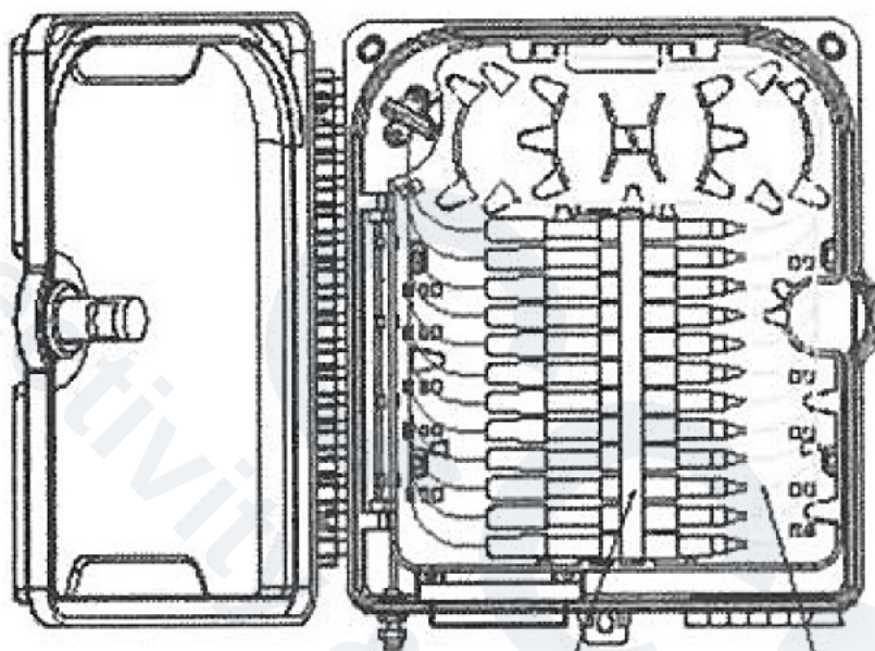
Supporto per 12 bussole SC/LC Duplex 12 SC/LC Duplex adapters holder
