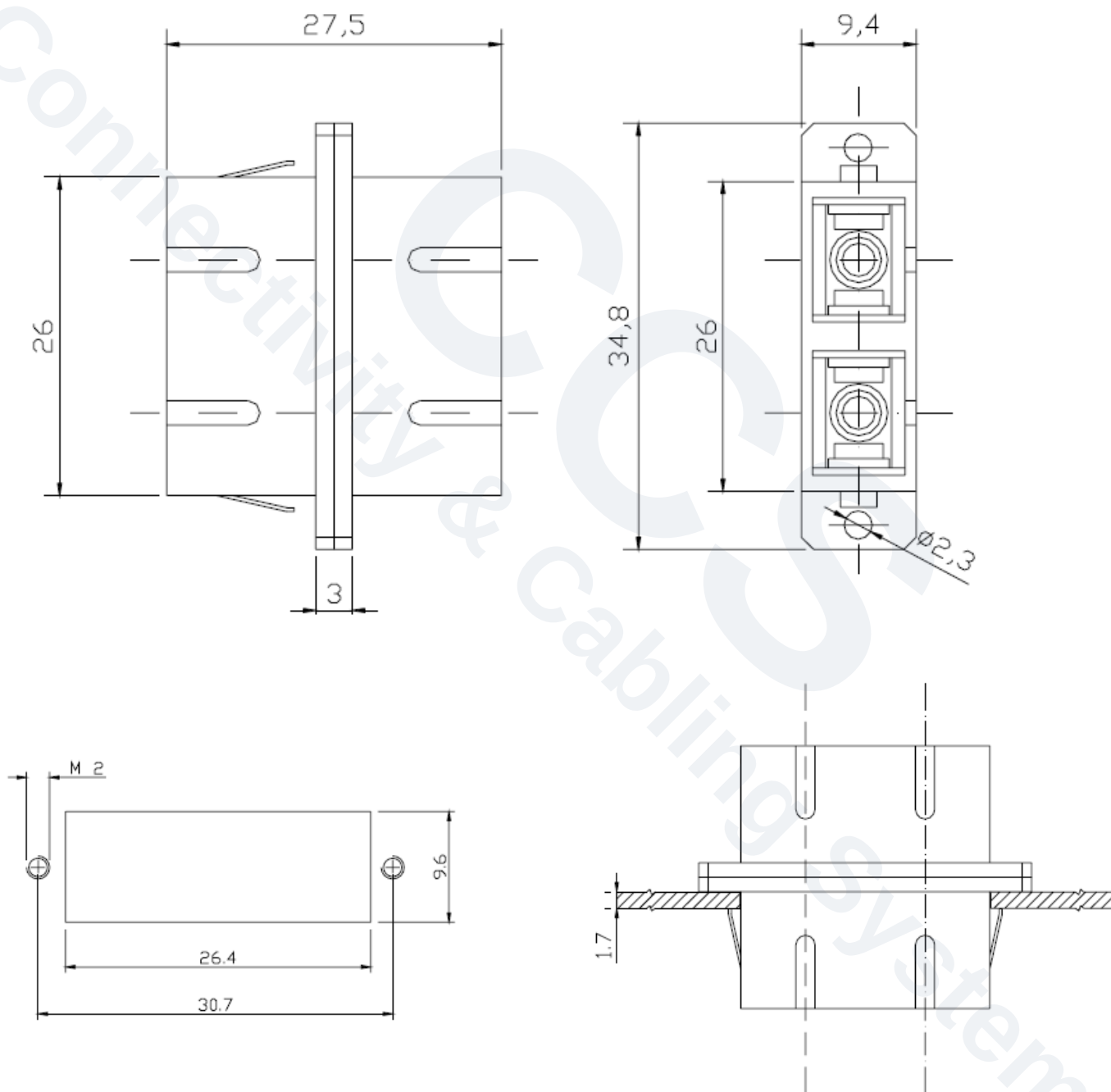
Fori sul pannello/Panel hole
